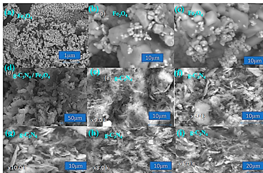
FIGURE 3 SEM micrographs of (A–C) \text{Fe}_3\text{O}_4 , (D) \text{g-C}_3\text{N}_4/\text{Fe}_3\text{O}_4 , and (E–I) \text{g-C}_3\text{N}_4 .
