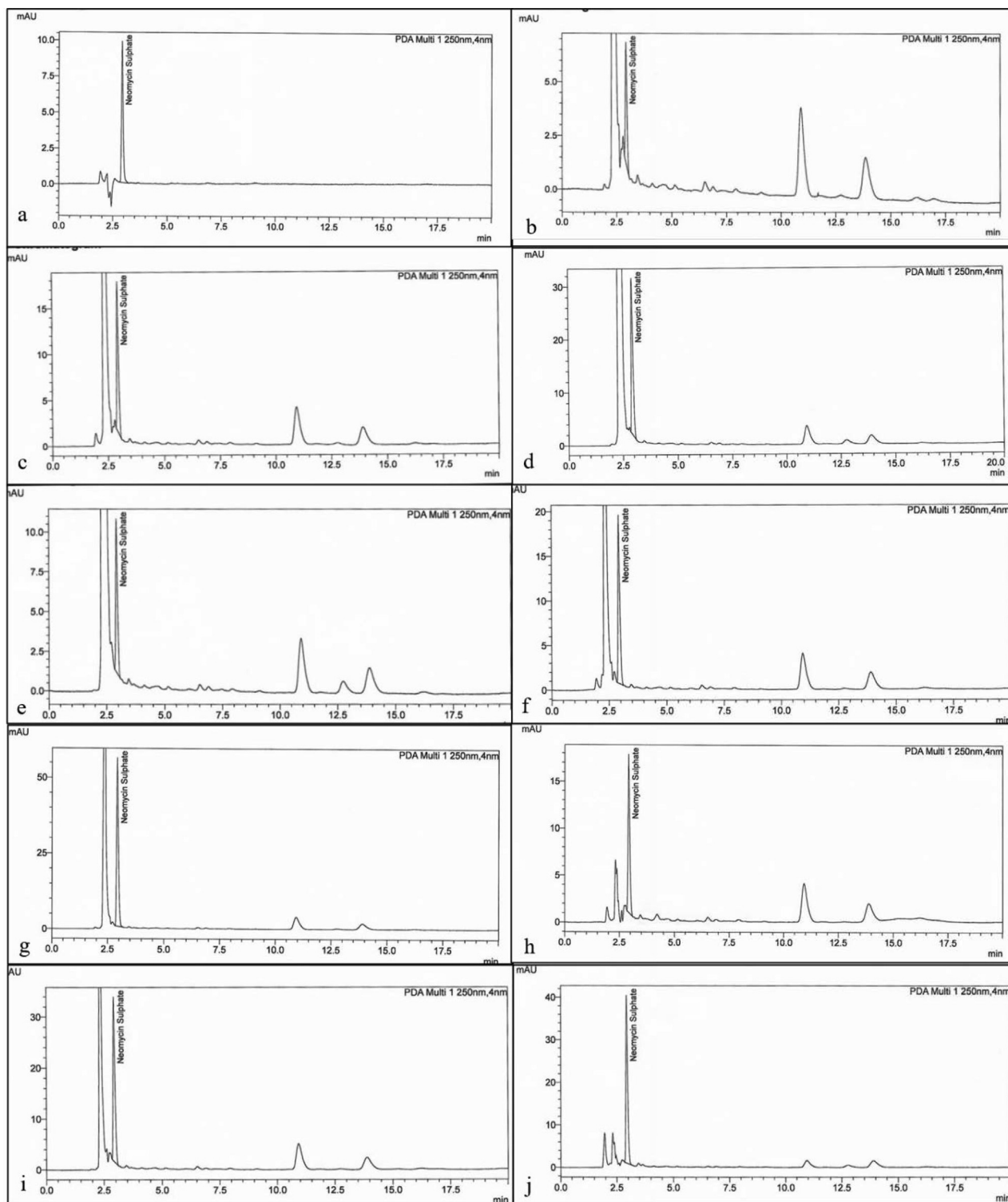
Fig. 2. HPLC-UV of a) Neomycin sulphate standard, b) NE-1, c) NE-2, d) NE-3, e) NE-4, f) NE-5, g) NE-6, h) NE-7, i) NE-8 and j) NE-9.
